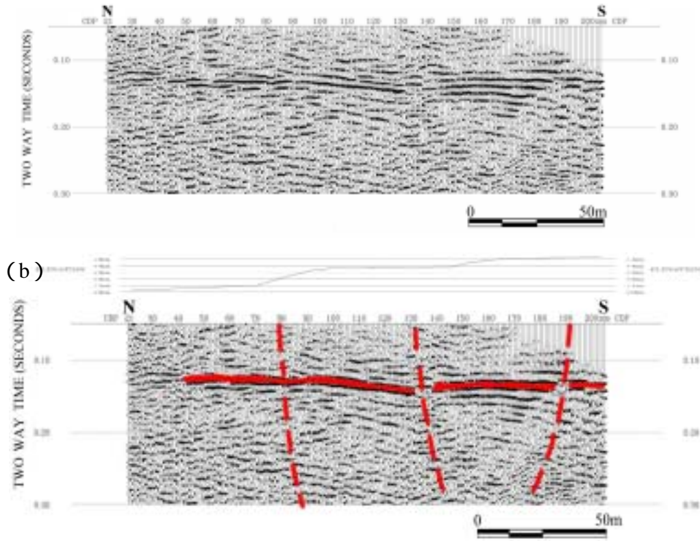
圖二 測線 00P-SHF-SH-C 之重合剖面(a)及其解釋(b)。
