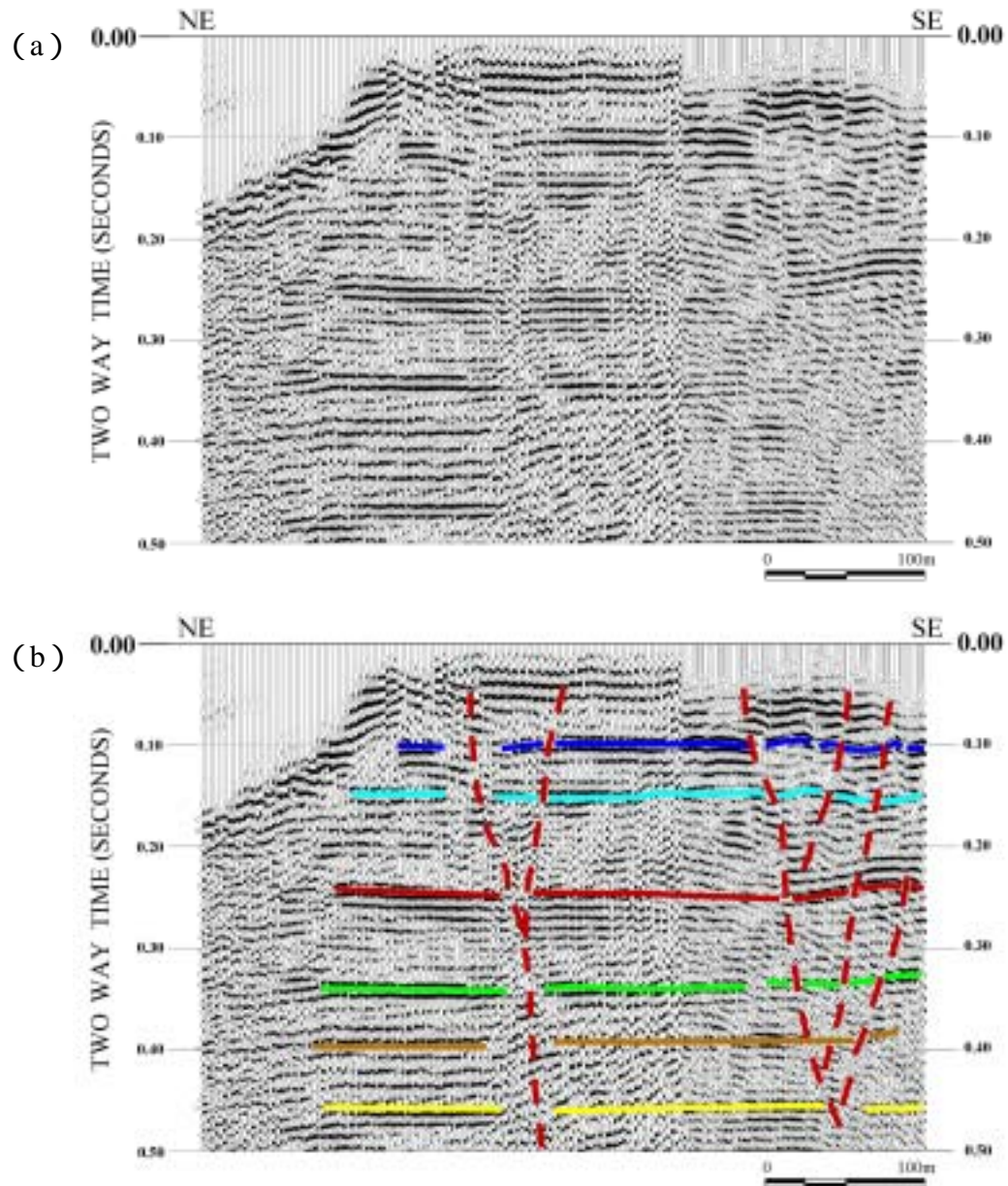
圖五 測線 02P-SHF-SH-B 之重合剖面(a)及其解釋(b)。
