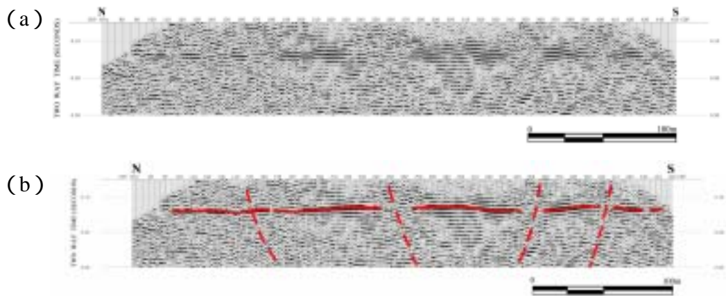
圖三 測線 97P-SHF-SH-A 之重合剖面(a)及其解釋(b)。
